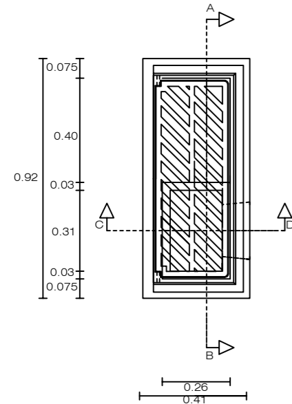
EMBORNAL TIPUS BADALONA
