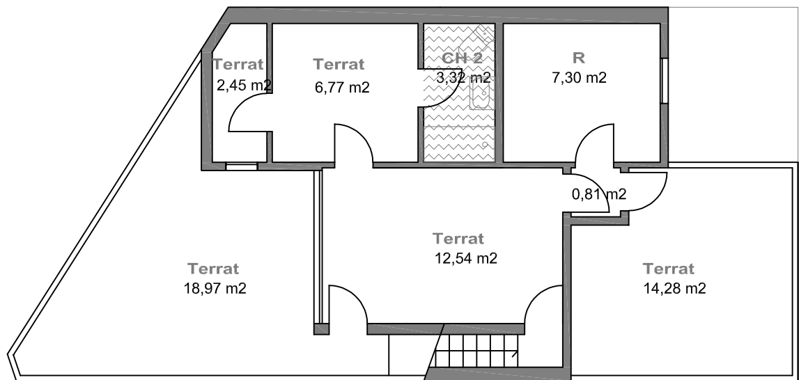
PLANTA COBERTA
