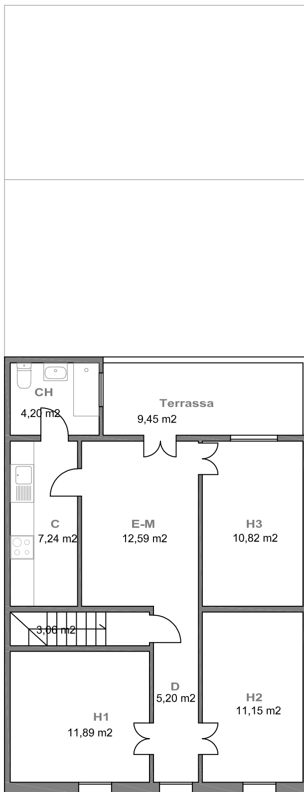
PLANTA PIS
