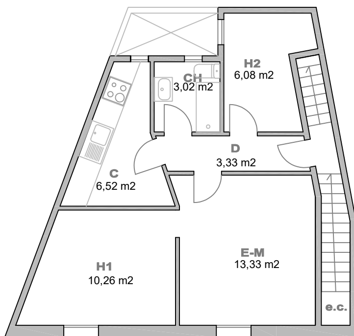
PLANTA PRIMERA
