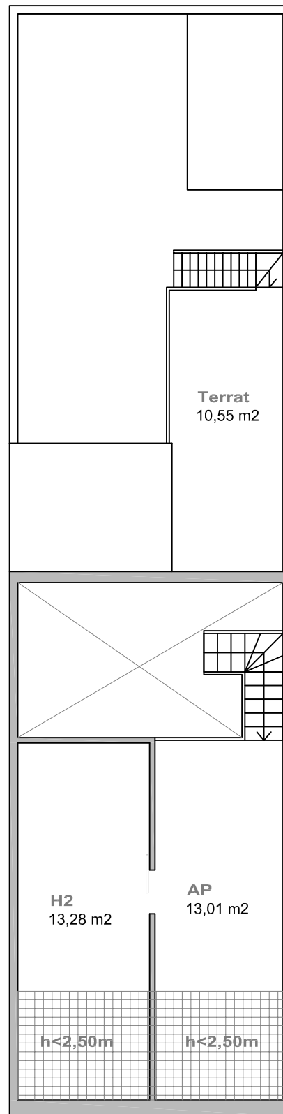
PLANTA ALTELL
