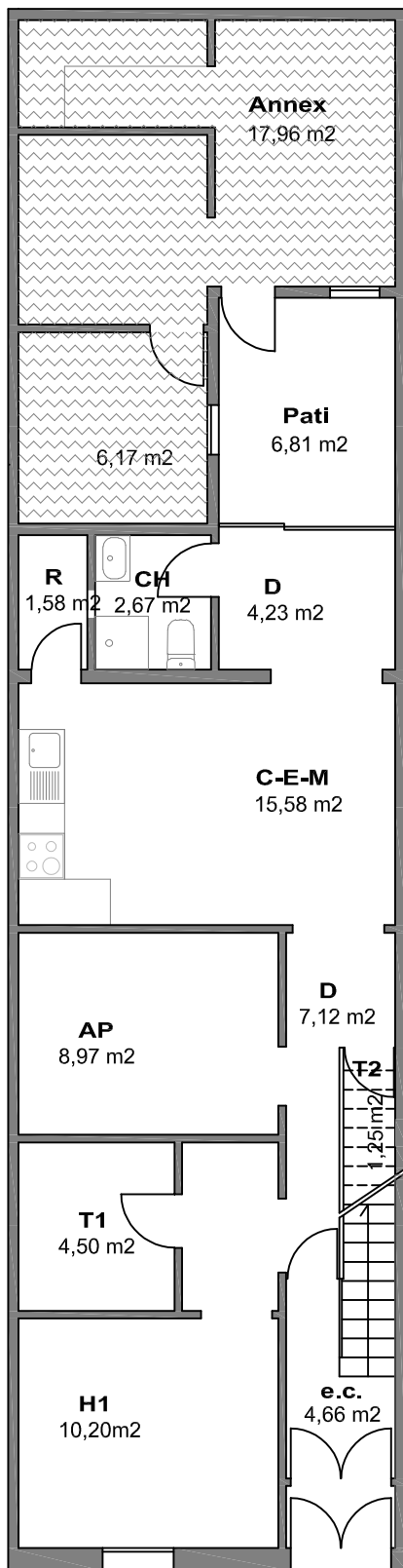
PLANTA BAIXA
