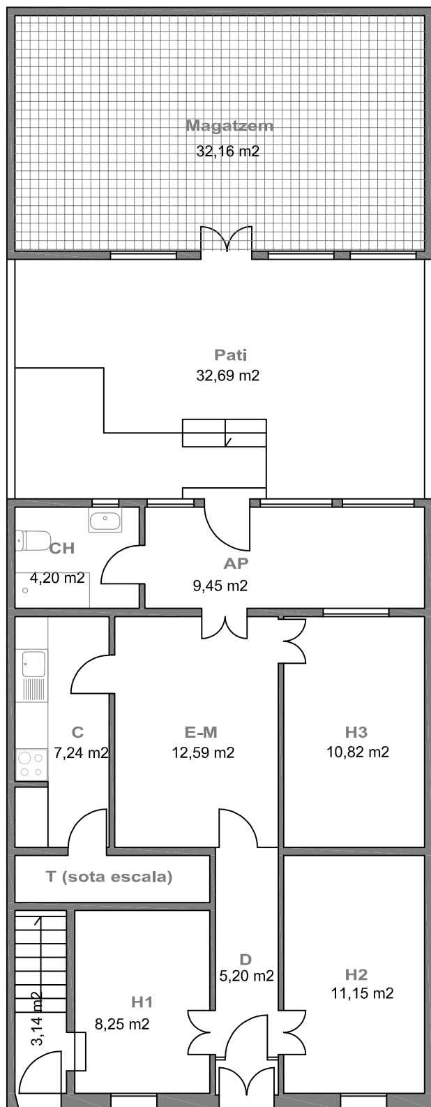
PLANTA BAIXA
