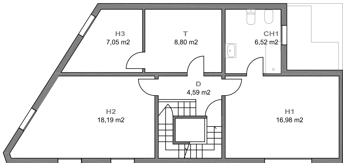
PLANTA PRIMERA
