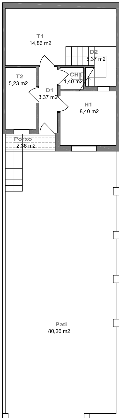
PLANTA BAIXA
