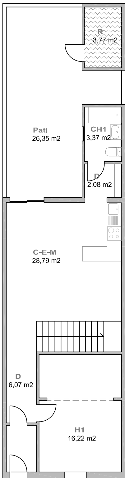
PLANTA BAIXA
