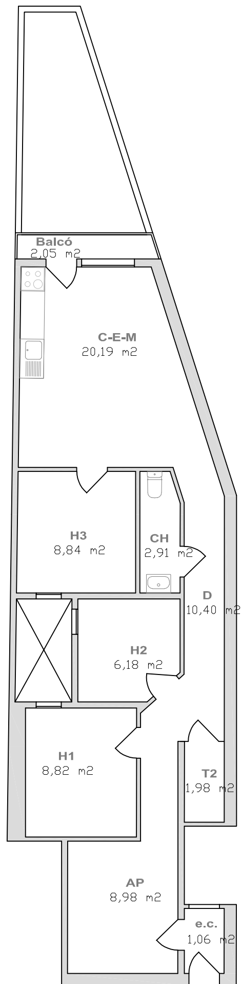
PLANTA BAIXA
