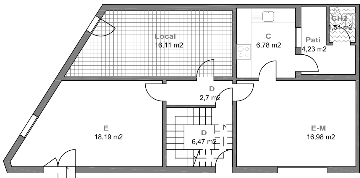
PLANTA BAIXA
