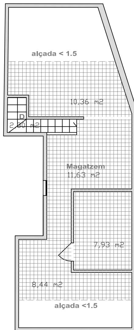
ALTELL (sotacoberta)
