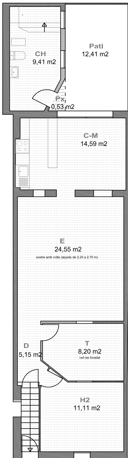
PLANTA SOTERRANI
