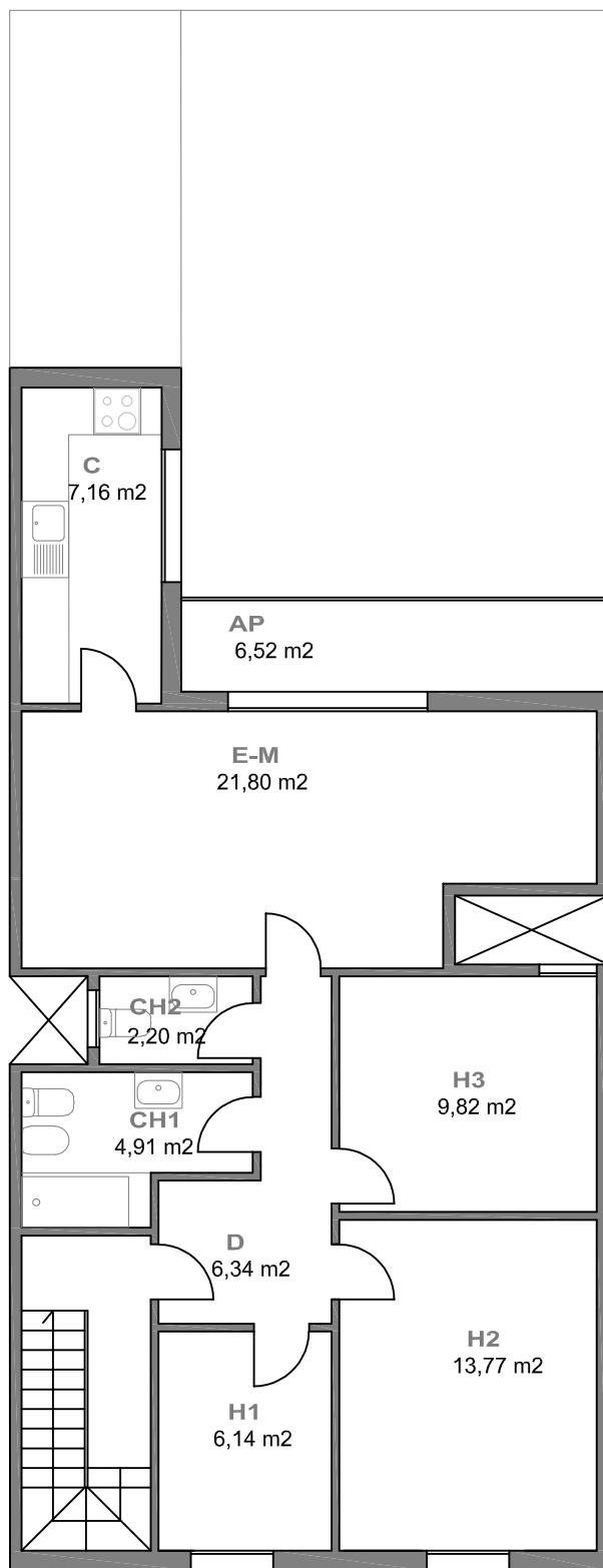
PLANTA TERCERA
