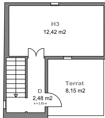
ALTELL
