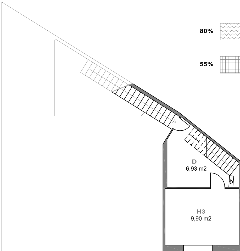
PLANTA PIS
