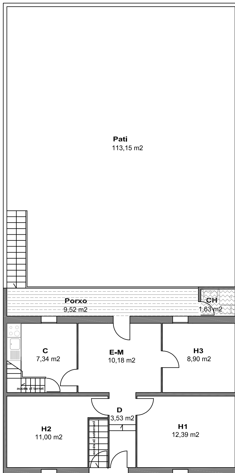
PLANTA BAIXA
