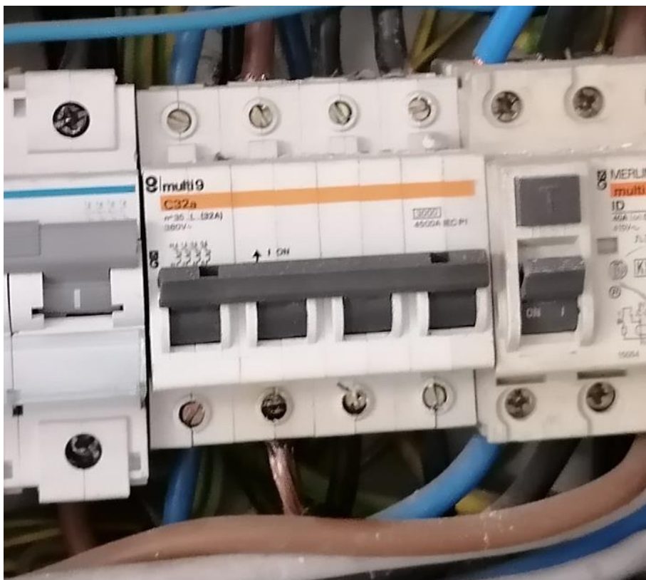
Imatge 7 – connexions a proteccions incorrectes
