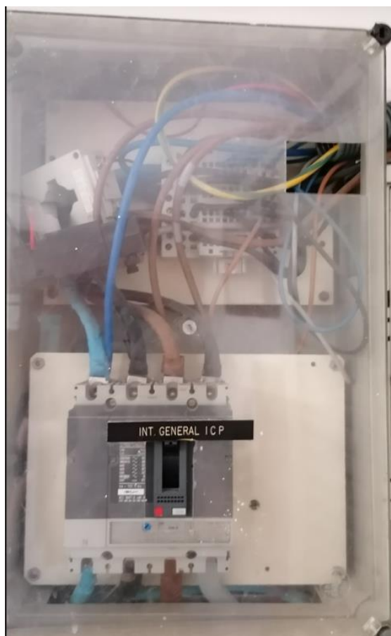
Imatge 6 – cablejat sobre ICP
