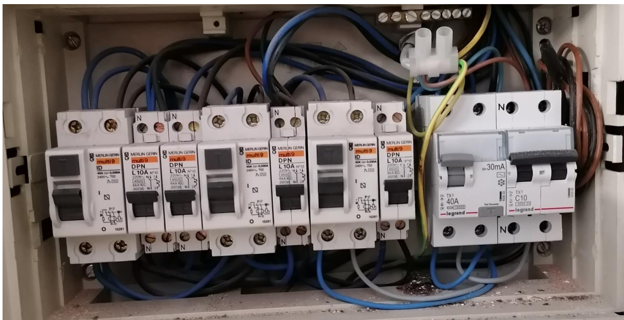
Imatge 5 – connexions en punta i encintades dins del quadre
