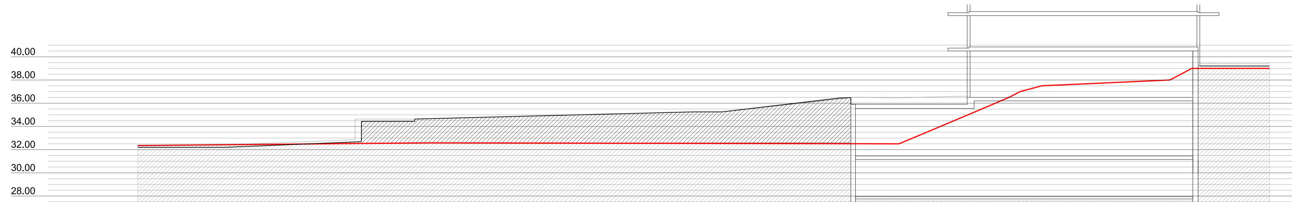
PERFIL 9 TERRES APORTADES 131.50 m 2
