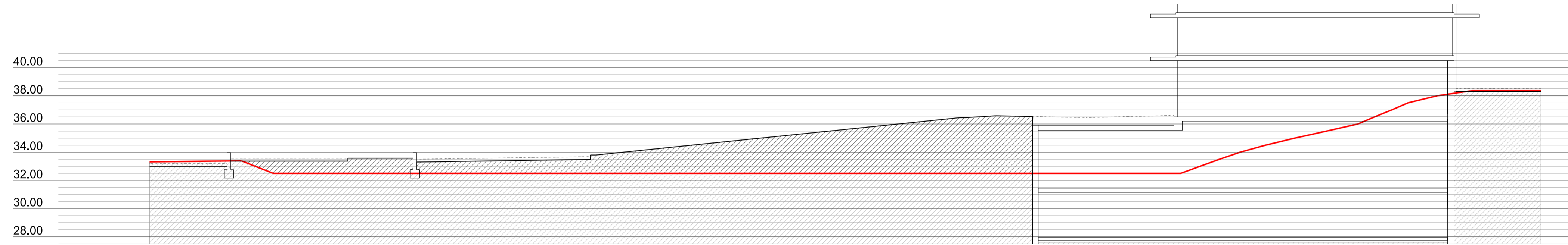
PERFIL 7 TERRES APORTADES 123.70 m 2
