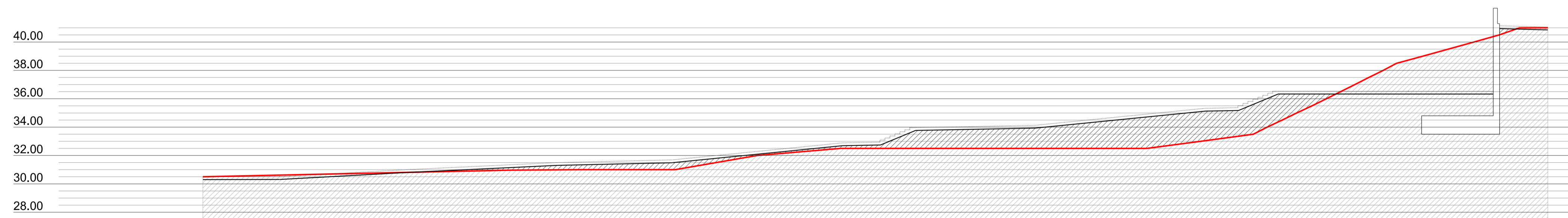
PERFIL 13 TERRES APORTADES 58.50 m 2 EXCAVACIÓ 26.00 m 2
