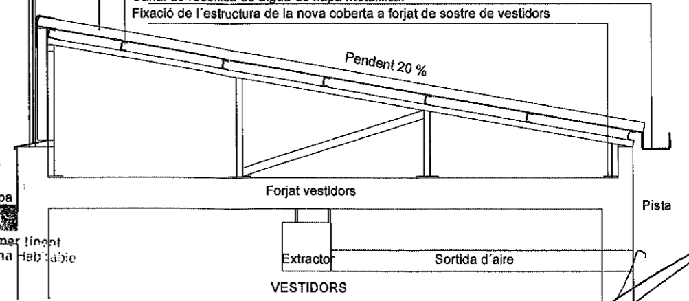
SECCIÓ DETALL COBERTA
