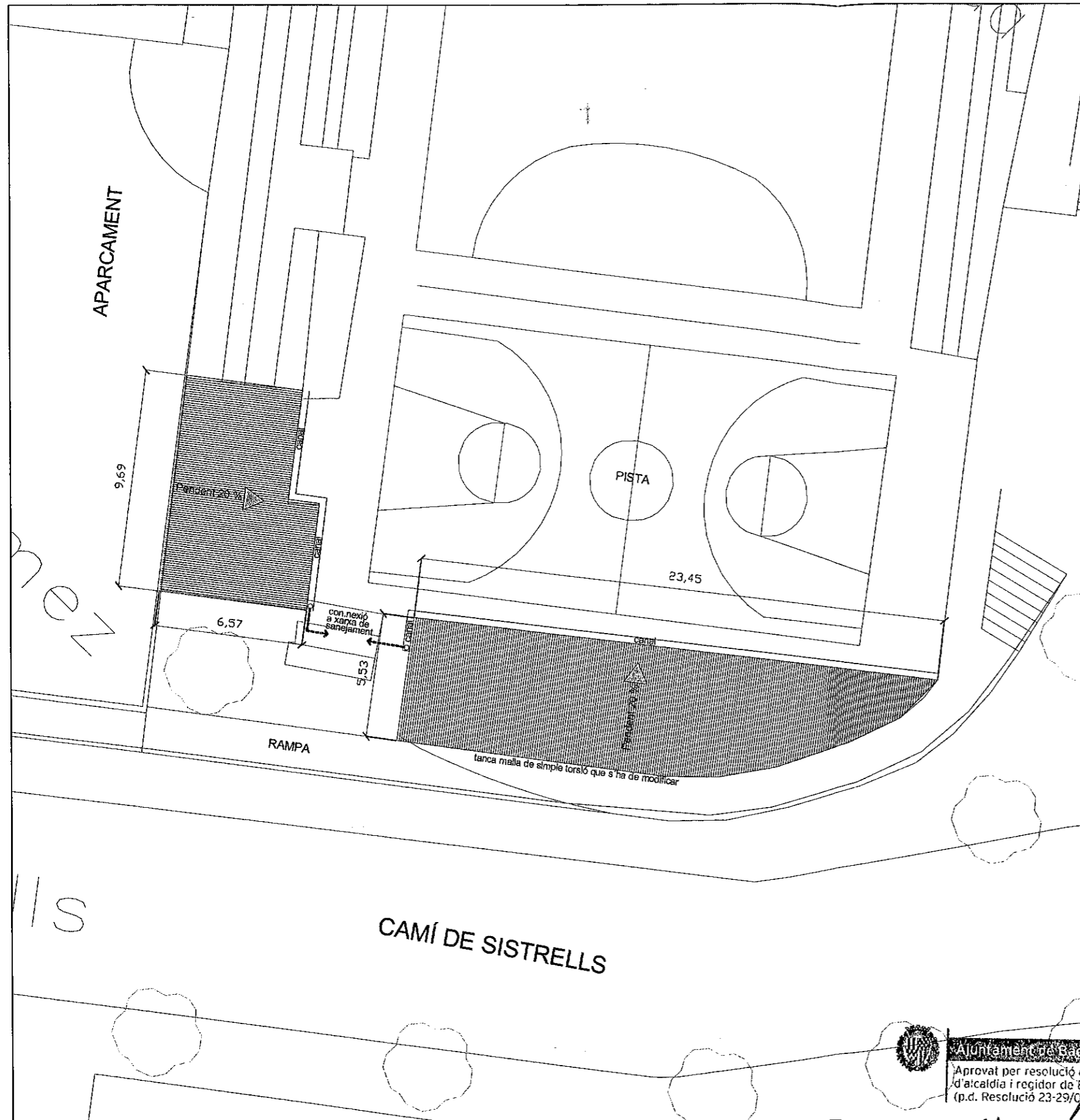
PLANTA GENERAL
