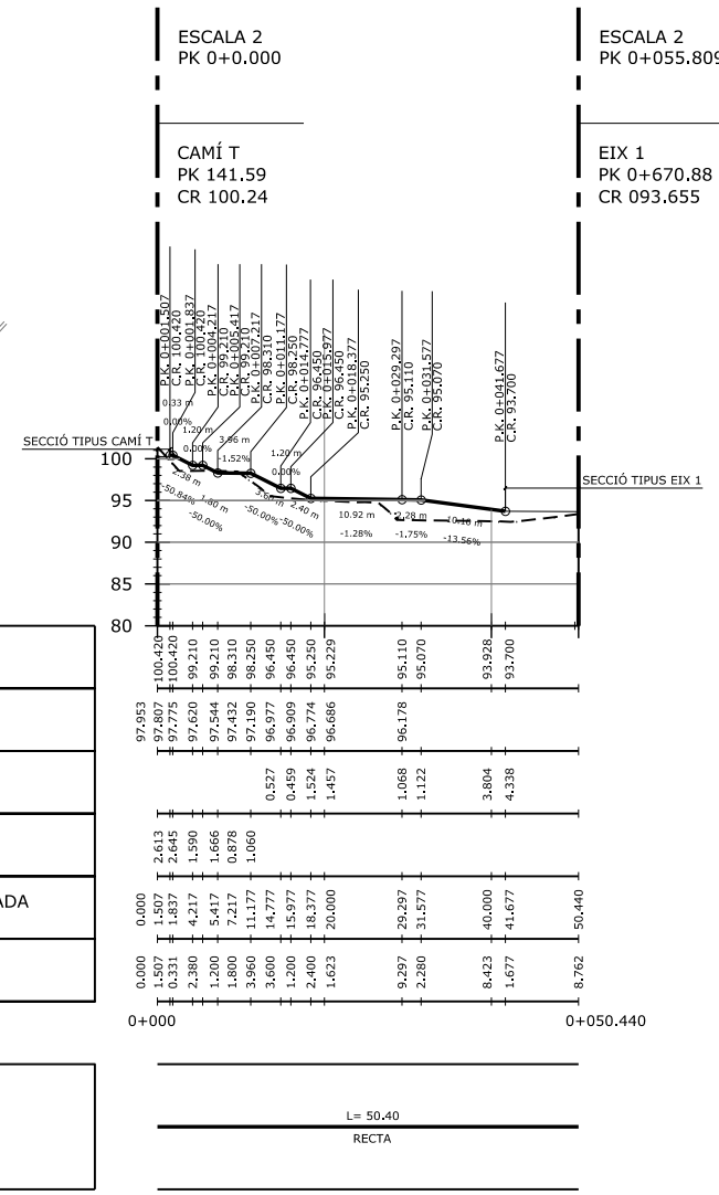
PERFIL LONGITUDINAL ESCALA 2 P.K. 0+000,000 A P.K. 0+050.440 ESCALA DIN A-1 H=1:500 I V=1:500 ESCALA DIN A-3 H=1:1000 I V=1:1000
