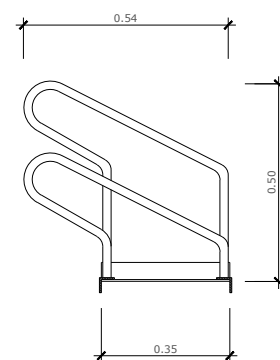
SECCIÓ ESCALA DIN A-1: 1/10 ESCALA DIN A-3: 1/20
