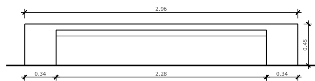
VISTA FRONTAL ESCALA DIN A-1: 1/20 ESCALA DIN A-3: 1/40
