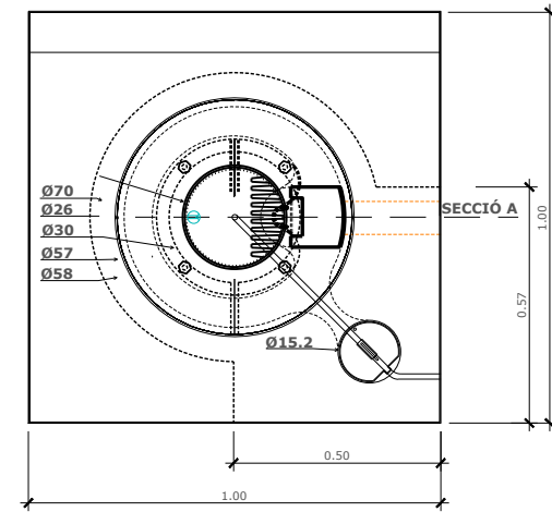
PLANTA ESCALA DIN A-1: 1/10 ESCALA DIN A-3: 1/20
