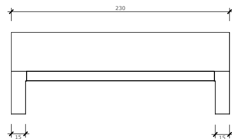
VISTA FRONTAL ESCALA DIN A-1: 1/20 ESCALA DIN A-3: 1/40
