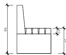
VISTA LATERAL ESCALA DIN A-1: 1/20 ESCALA DIN A-3: 1/40
