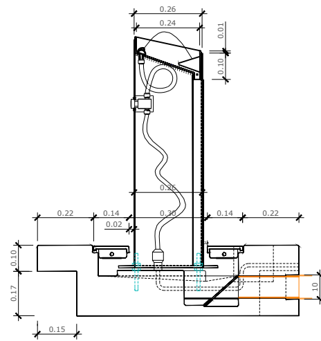
SECCIÓ A ESCALA DIN A-1: 1/10 ESCALA DIN A-3: 1/20
