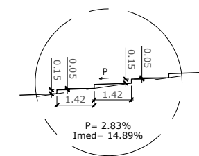
DETALL FORMACIÓ RAMPA ITALIANA CAMÍ C ESCALA 1:100
