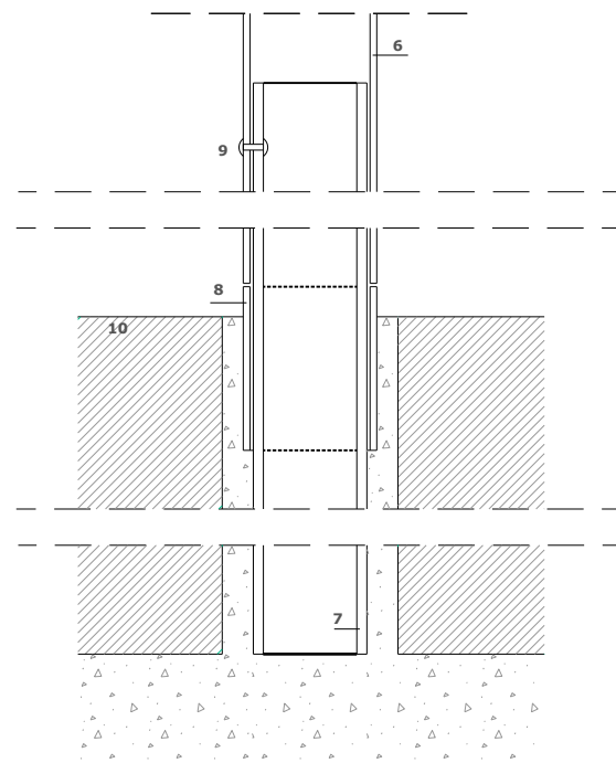
DETALL ANCORATGE
