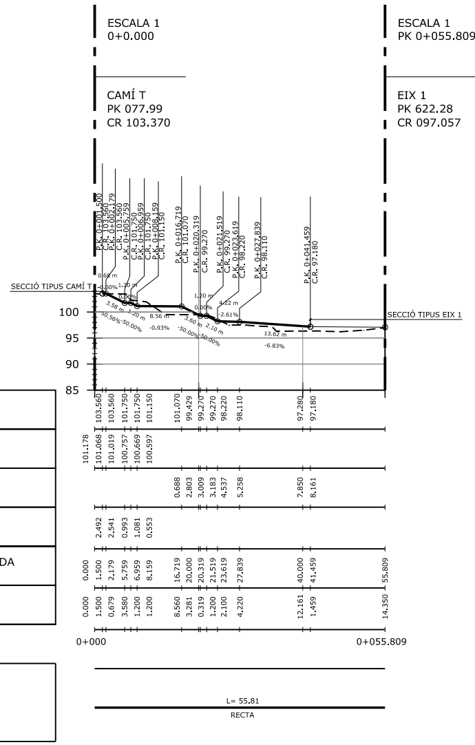
PERFIL LONGITUDINAL ESCALA 1 P.K. 0+000,000 A P.K. 0+055.809 ESCALA DIN A-1 H=1:500 I V=1:500 ESCALA DIN A-3 H=1:1000 I V=1:1000
