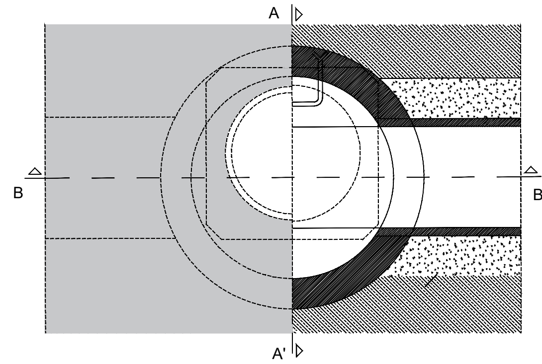
POU DE REGISTRE CIRCULAR A CALÇADA
