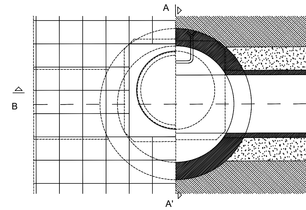
SECCIÓ A-A' TRANSVERSAL POU PASSANT
