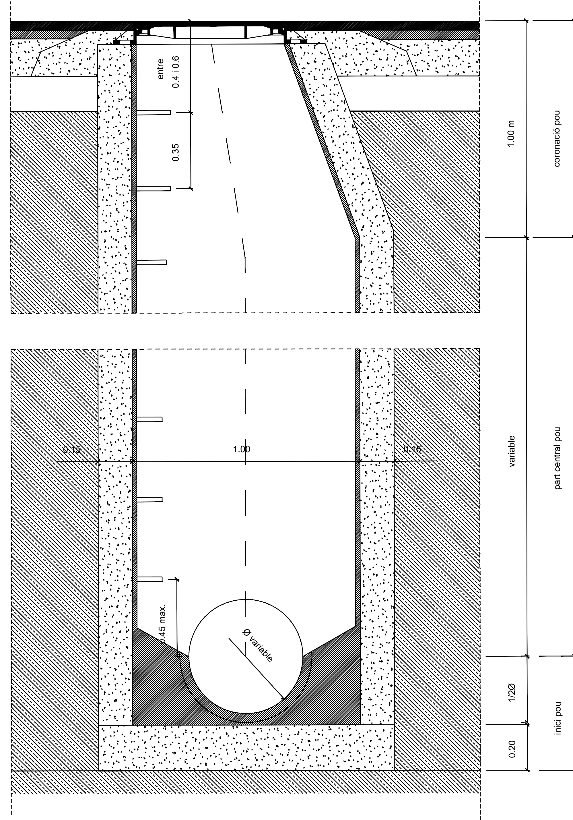
SECCIÓ A-A' TRANSVERSAL POU PASSANT
