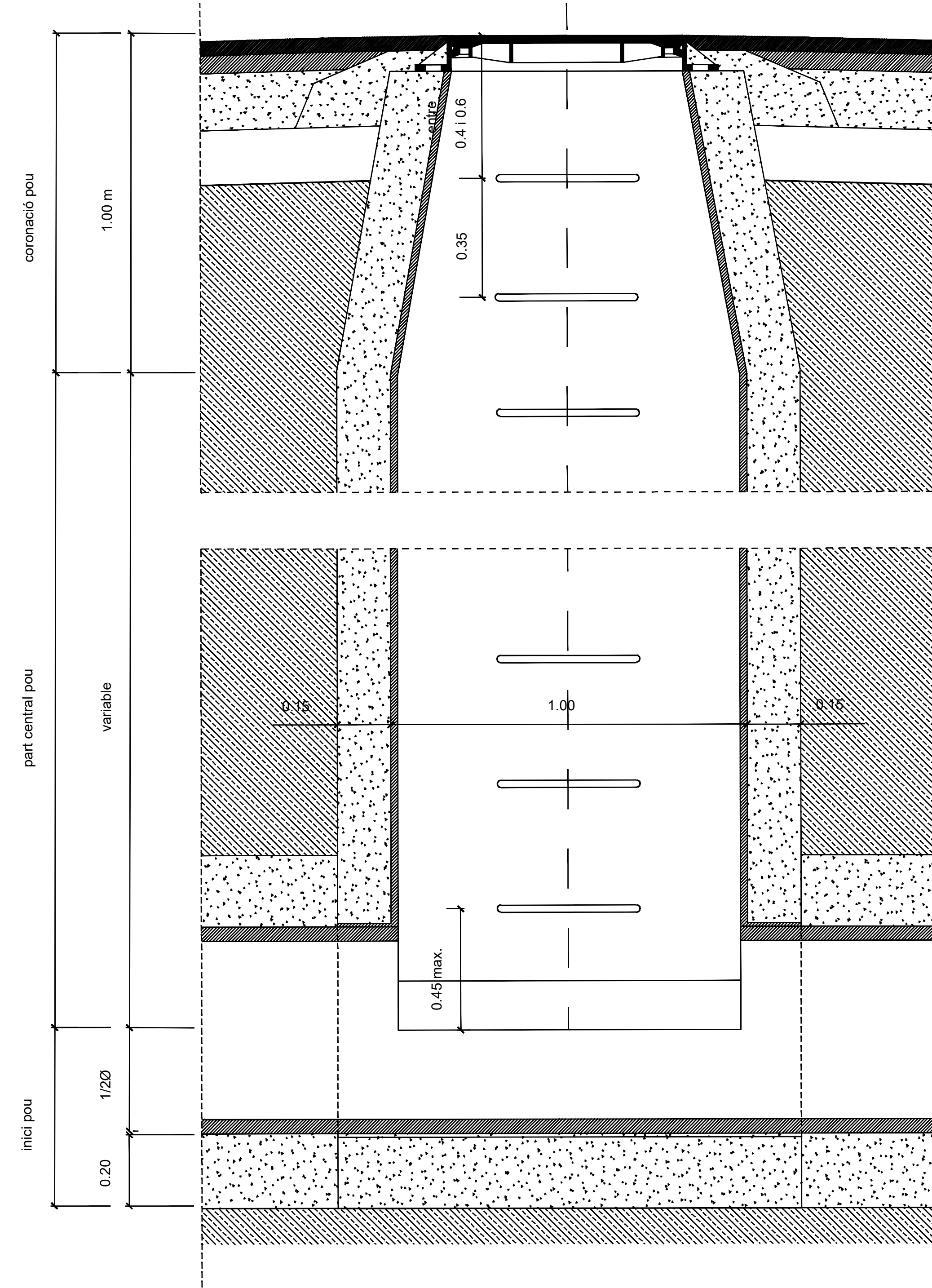
SECCIÓ B-B' LONGITUDINAL POU PASSANT
