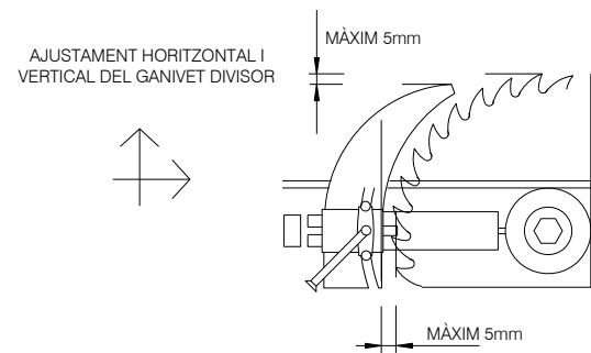
GANIVET DIVISOR
