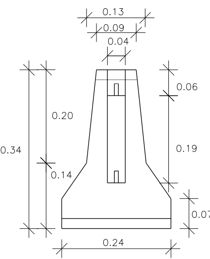
ALÇAT TRANSVERSAL
