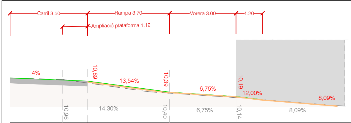
SECCIÓ A-A' ESCALA 1/100
