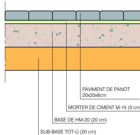
SECCIÓ VORERA AMB PANOT 20x20x8cm, COL·LOCACIÓ A TRUC DE MACETA ESCALA: 1/20
