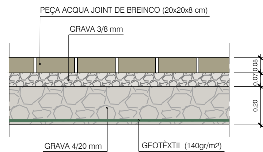
DETALL PAVIMENT DRENANT ESCALA: 1/20
