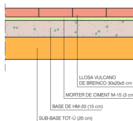
DETALL PAVIMENT LLOSA VULCANO ESCALA: 1/20
