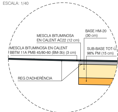
DETALL A ESCALA: 1/40
