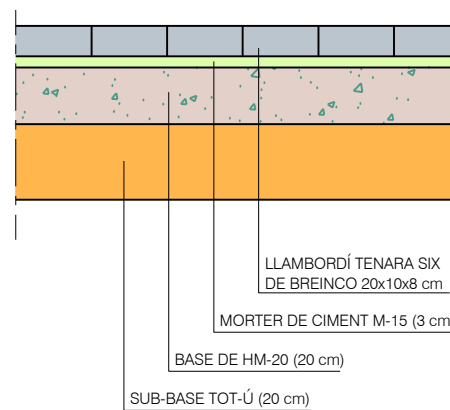
DETALL PAVIMENT DE LLAMBORDA TERANA SIX ESCALA: 1/20
