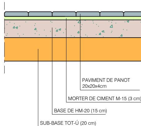
SECCIÓ VORERA AMB PANOT 20x20x4cm ESCALA: 1/20
