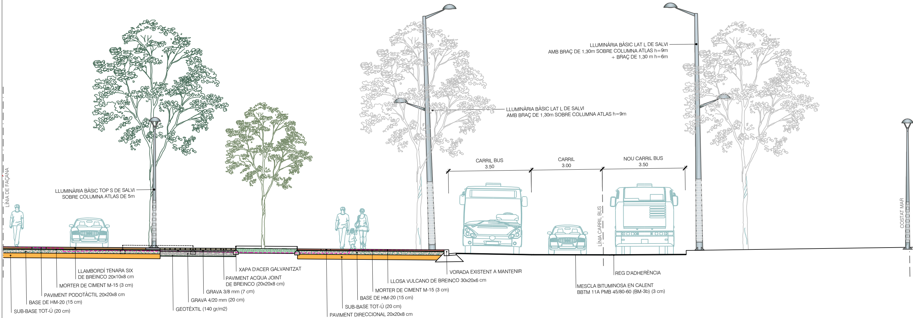
SECCIÓ S7 ESCALA: 1/100
