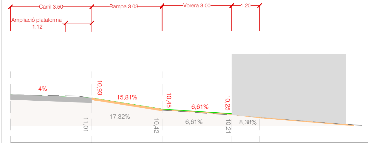
SECCIÓ B-B' ESCALA 1/100
