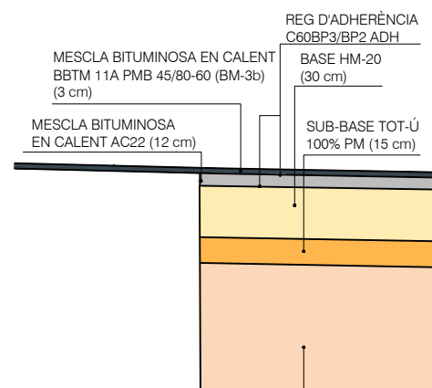
DETALL FERM AMPLIACIÓ CARRIL ESCALA: 1/40
