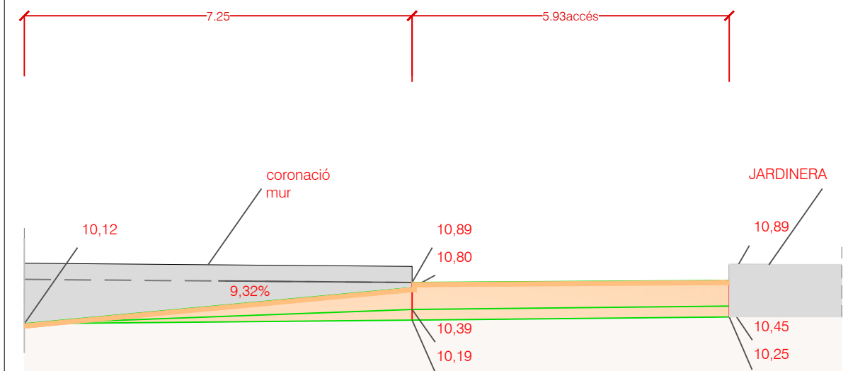
SECCIÓ C-C' ESCALA 1/100
