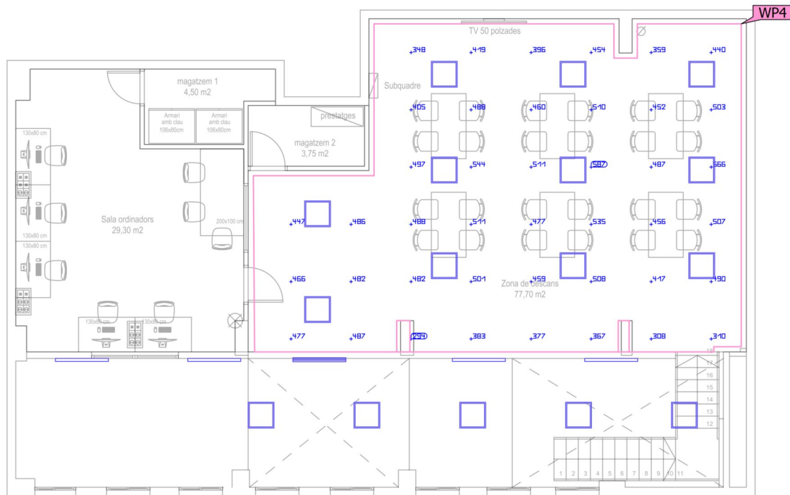
PLANTA ALTELL Proposta
